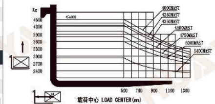
4.5T载荷曲线图 4.5T load curve
