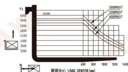
6.0T载荷曲线图
