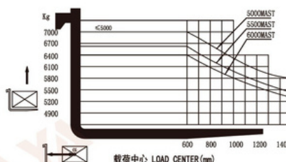
7.0T载荷曲线图
